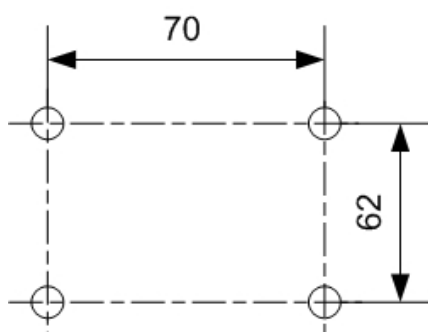
Расположение отверстий для крепления на основании ИПР-Р2
