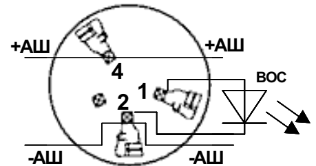
Рис. 1. Подключение базового основания серии В401 к адресной шине и к ВОС
