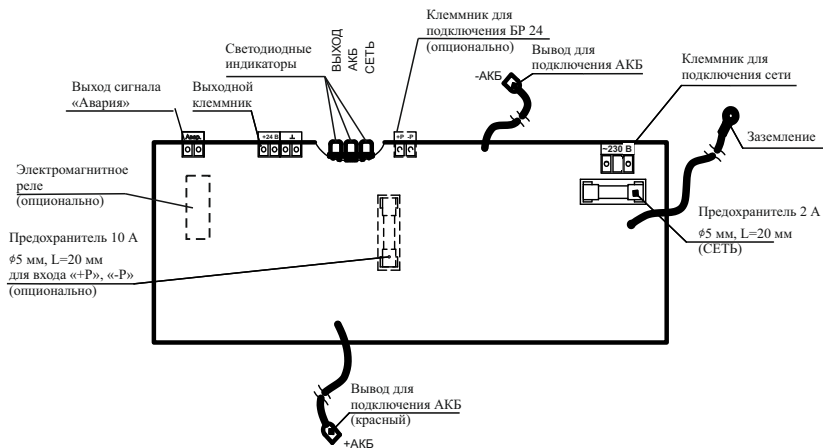
Рисунок 1 – Плата источника
