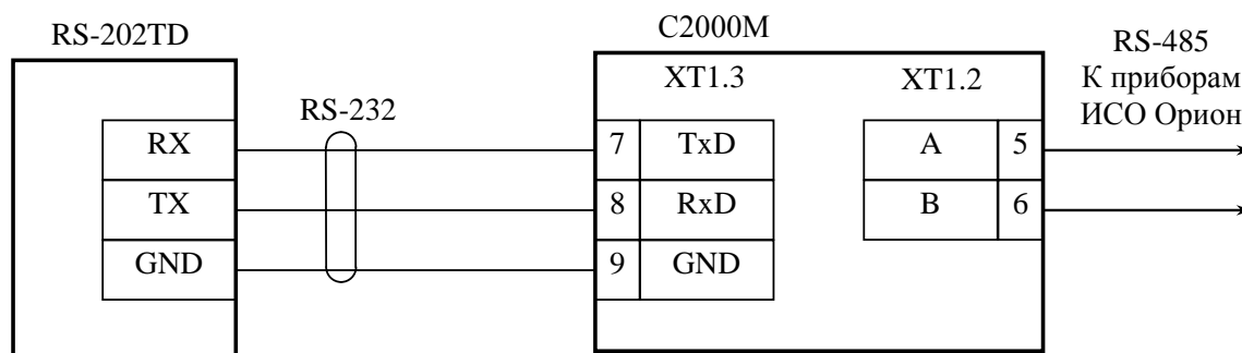
RS-202TD – радиопередатчик «Риф Стринг RS-202TD-RR»; C2000M - пульт контроля и управления «С2000М».
