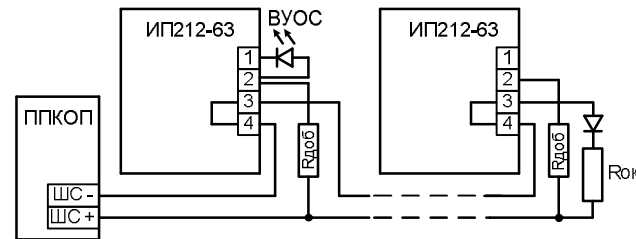
Рис.2 Типовая схема включения извещателя для приборов с переполюсовкой шлейфа сигнализации. Величина резисторов R_{ок} и R_{добр} определяется в соответствии с техническим описанием ППКОП
